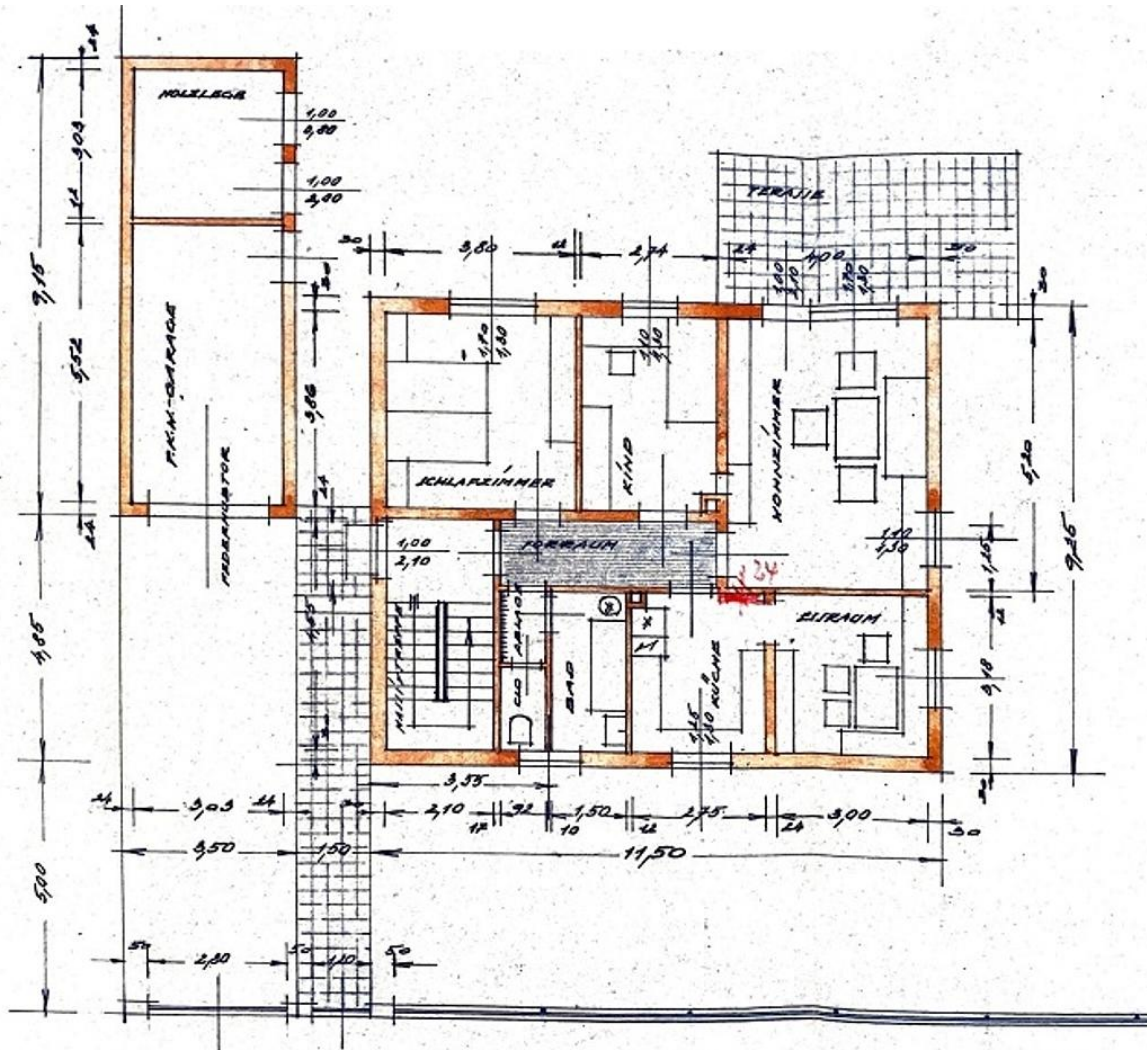
ERDGECHOSSGRUNDRISS 1:100
