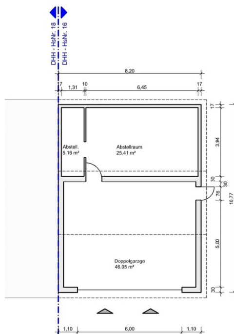
GRUNDRISS - DOPPELGARAGE
