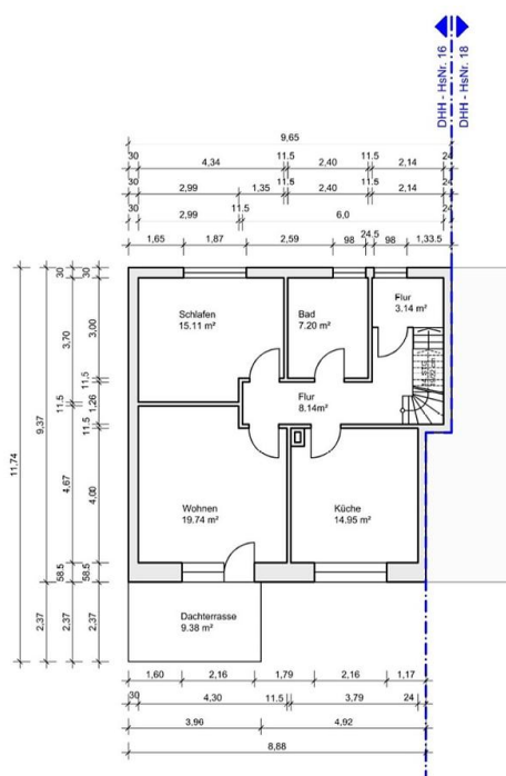
OBERGESCHOSS
